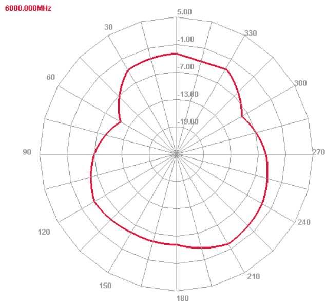
6000MHz H Plane
