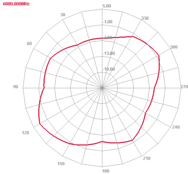
6000MHz E Plane
