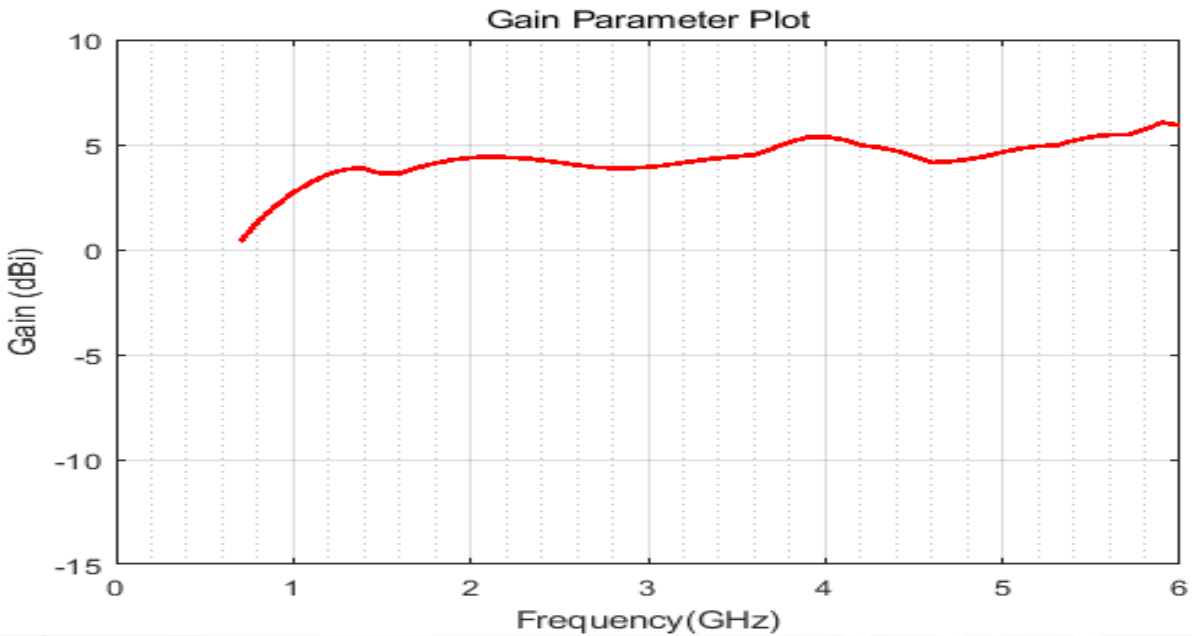
仿真天线增益曲线
