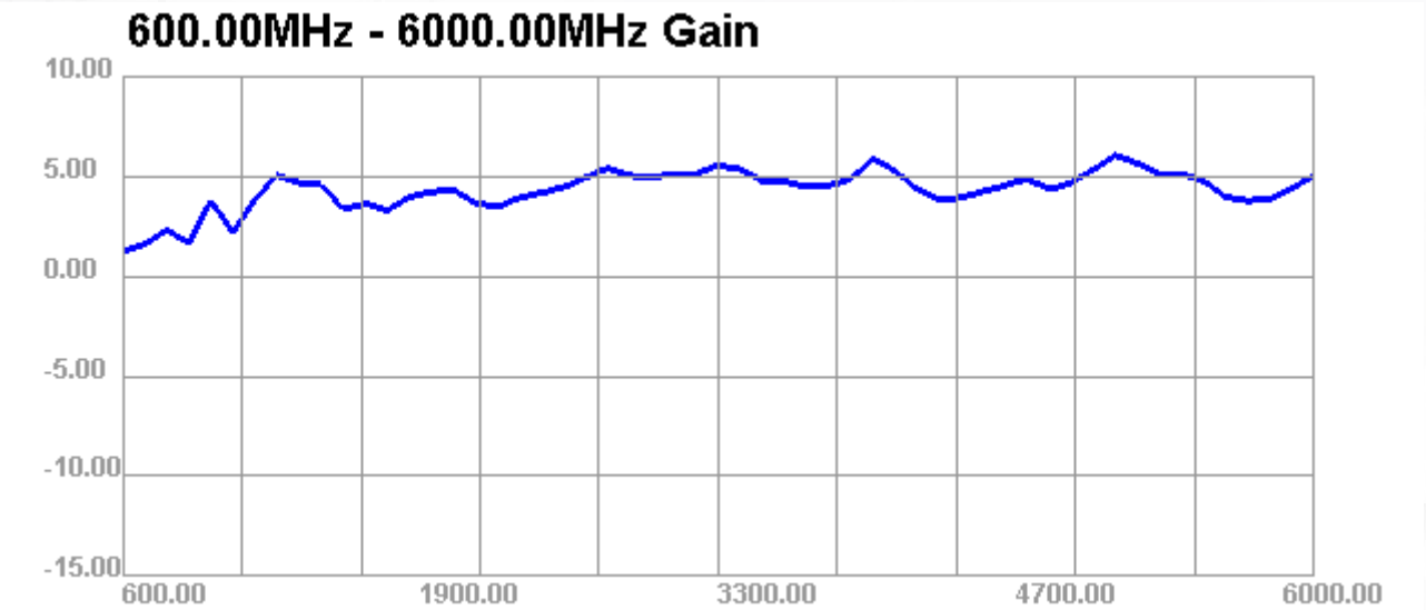
测量增益曲线
